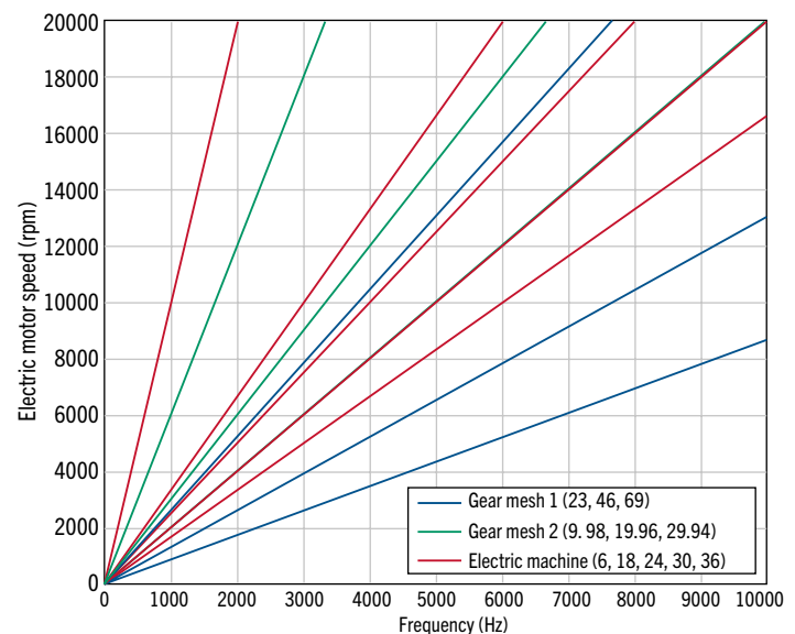
Fig. 1 - Diagramma di Campbell per la EDU studiata
