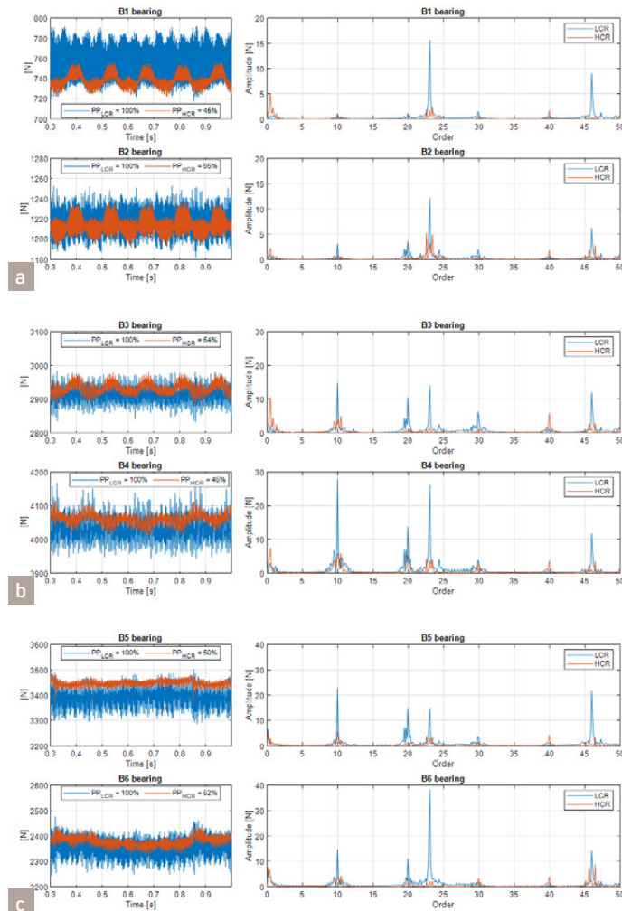
Fig. 13 - Forze sui cuscinetti FM - scatola flessibile
